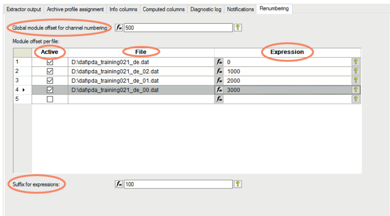
Fig. 9: Renumbering tab
